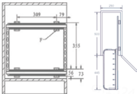
ESQUEMA INSTALACIÓN ORGANIZADOR WISCONSIN
