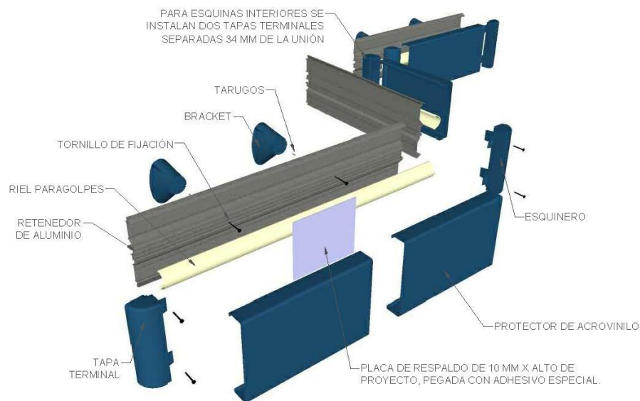
TERMINACIÓN ESQUINA INTERIOR
