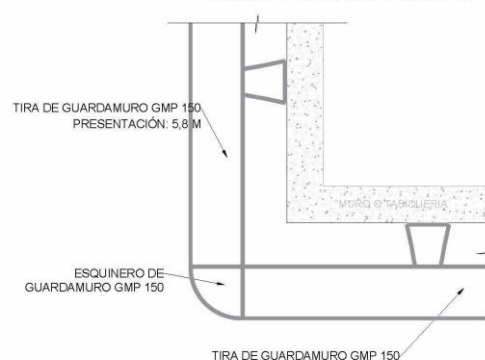
TERMINACIÓN ESQUINA EXTERIOR
