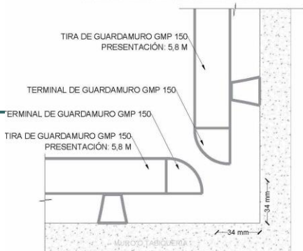
TERMINACIÓN ESQUINA INTERIOR
