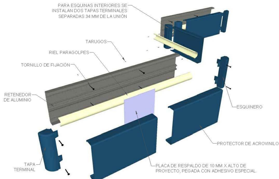
TERMINACIÓN ESQUINA INTERIOR
