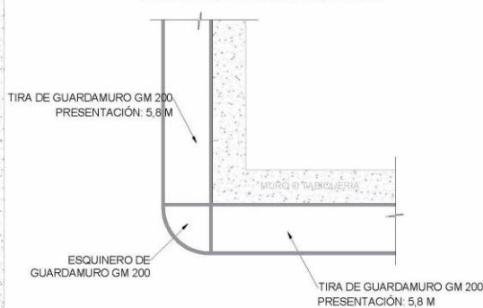
TERMINACIÓN ESQUINA EXTERIOR
