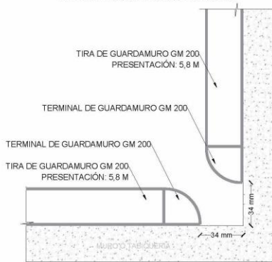
TERMINACIÓN ESQUINA INTERIOR
