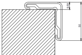
VISTA PERFIL
