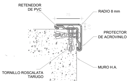
VISTA CORTE
