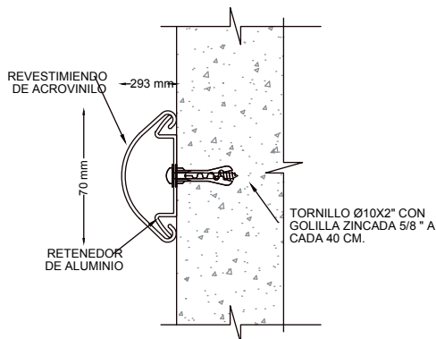
VISTA CORTE
